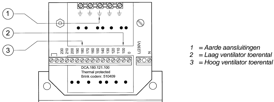
Figuur 5. Regeltransformator.
