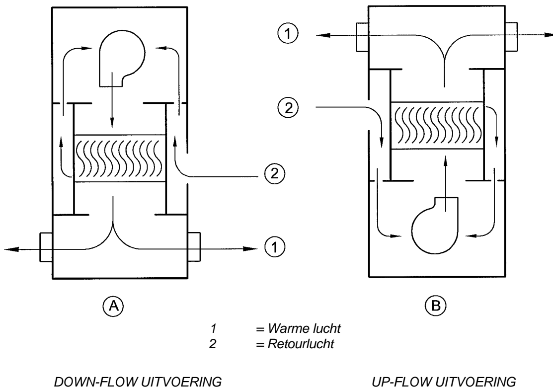
Figuur 1. Principeschets type.
