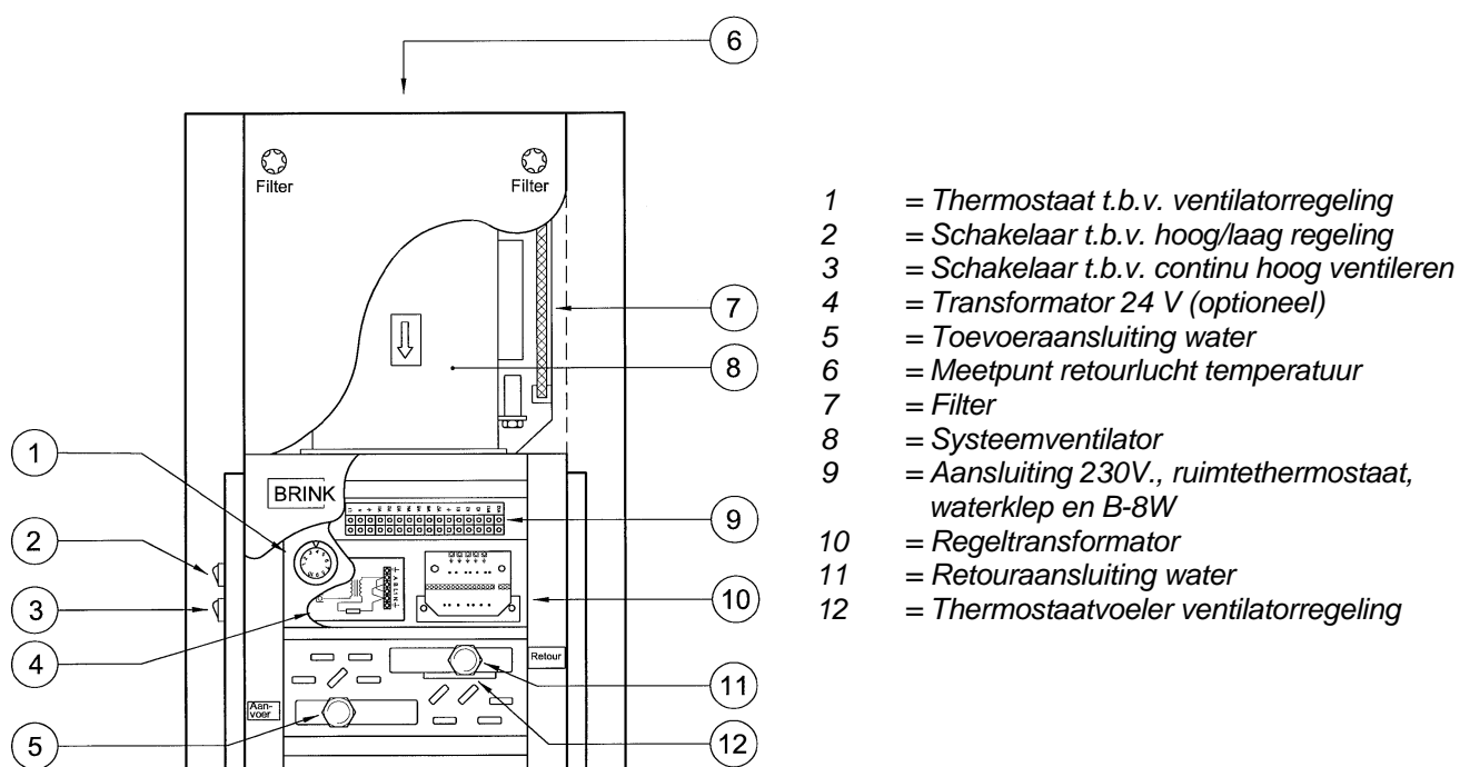
Figuur 2. Aanzicht bedieningsapparatuur B-8 IN-luchtverwarmer in Downflow uitvoering.
