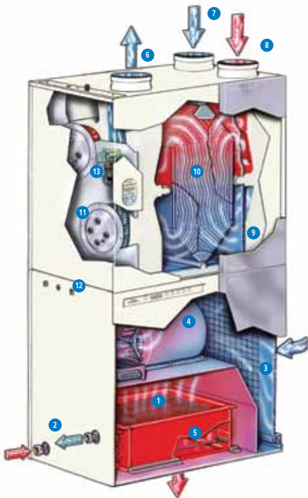
Afgebeeld is de rechteruitvoering van de Elan 10 Downflow met een Renovent HR 3b/1o
